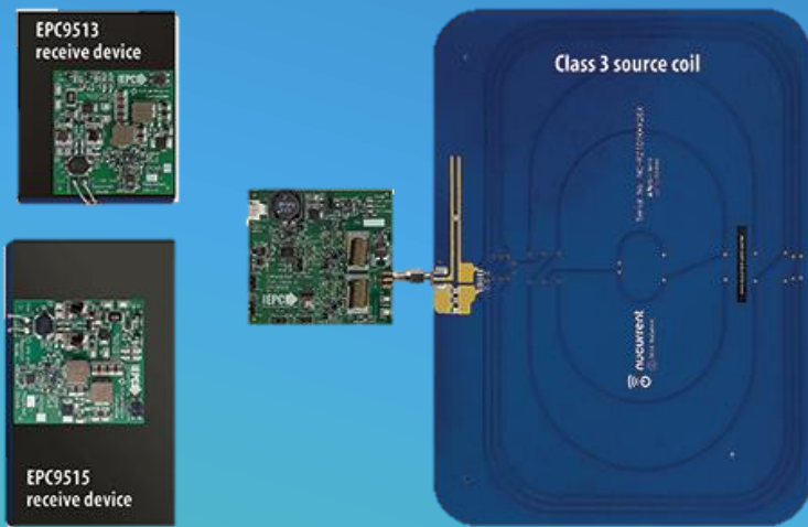
EPC9128, 16 Wクラス3のデモ・キット
