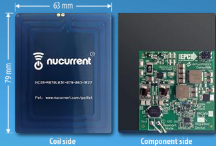
受電器EPC9513
